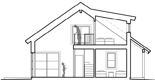
PRINCIPSNITT
