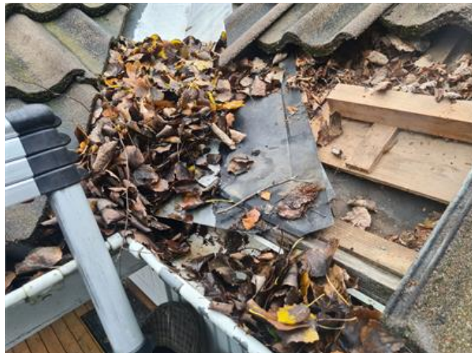
Tak, rikligt med löv i ränndal och hängrännor orsakat lokal fuktskada i takfot.
