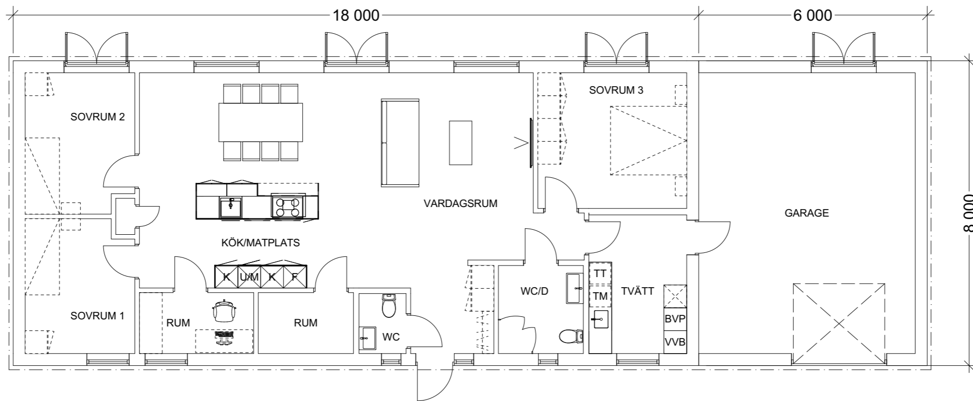
ENTRÉPLAN
