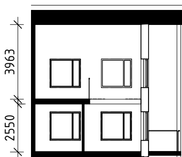
Sektion loft 1:200
