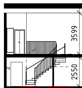
Sektion loft 1:200
