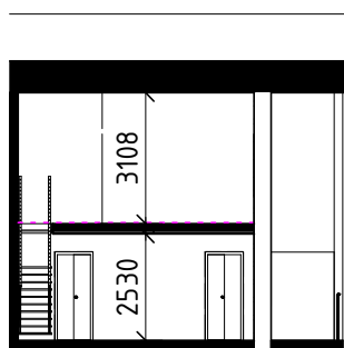
Sektion loft 1:200
