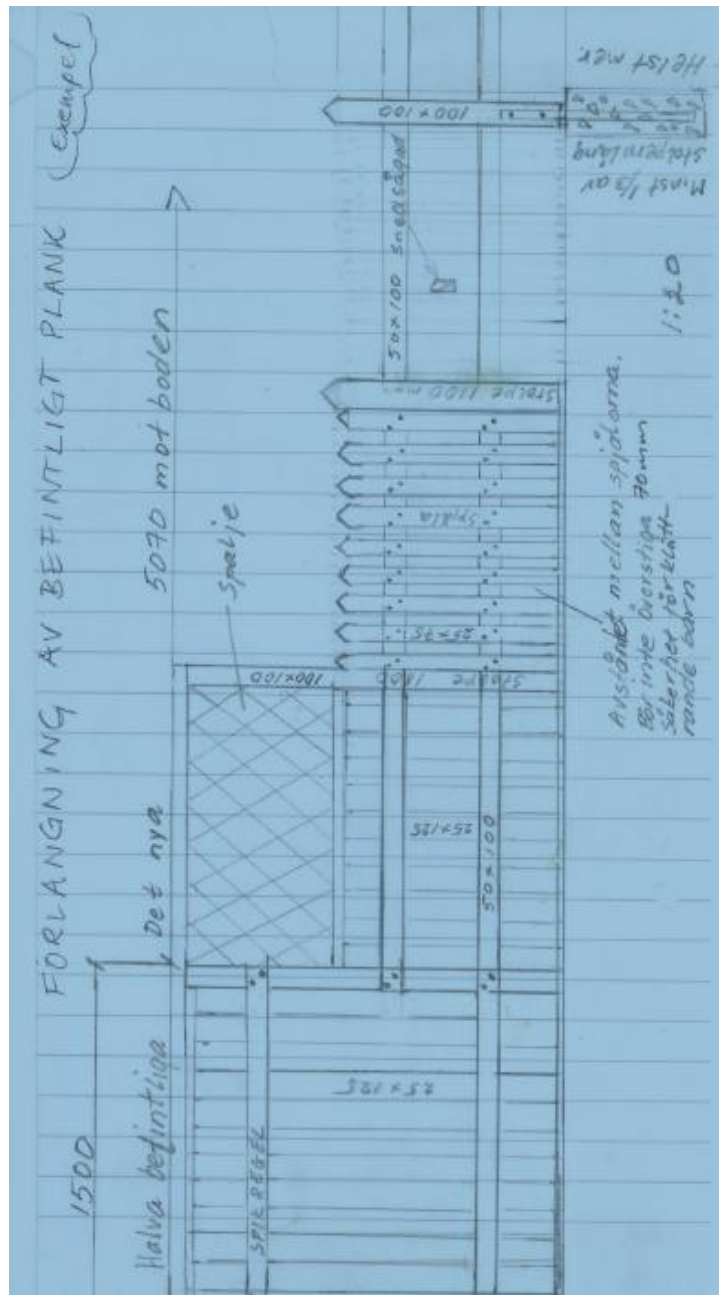
Bilaga: Exempel på staket mellan grannens tomt och din egen. Skala 1:20
