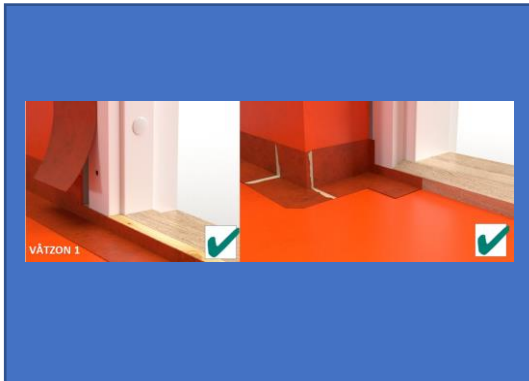
Bild 7: Godkänt montage, tätskikt mot tröskel.
