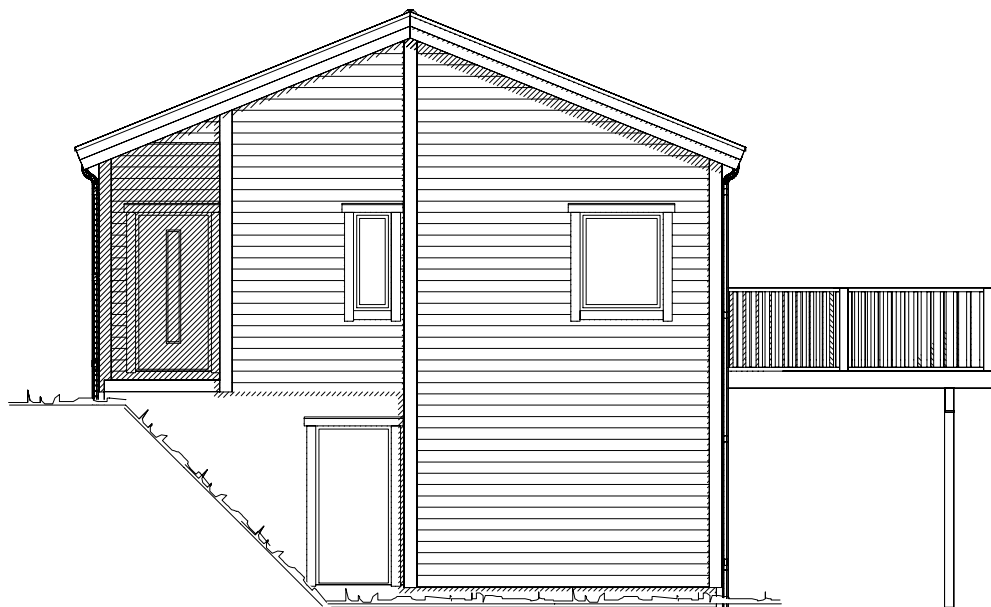
Fasad mot sydväst
