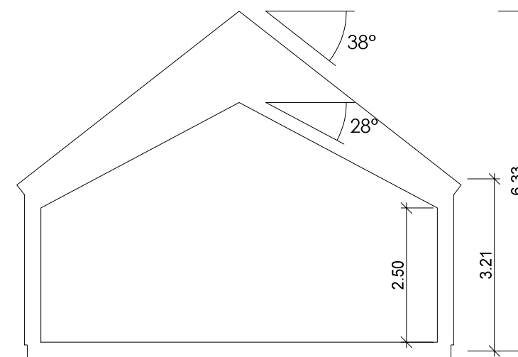
Sektion A-A
