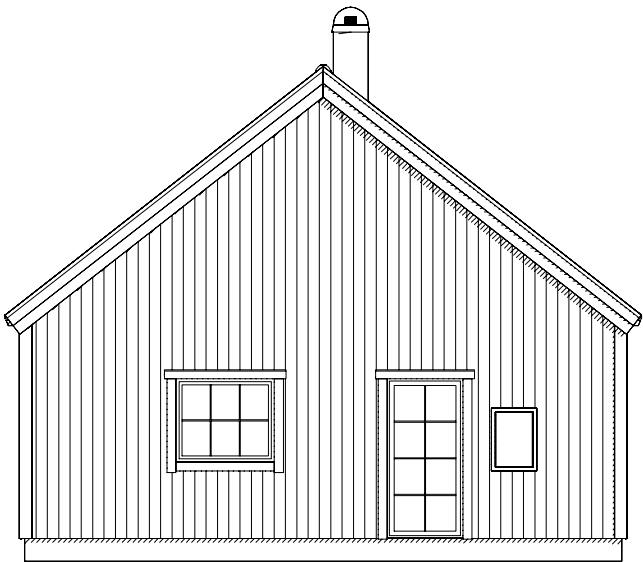
Fasad 4
