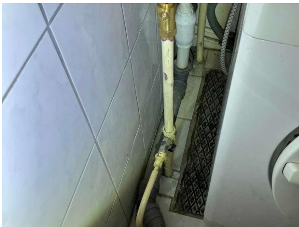
Bild 8: Invändigt, Entréplan, Tvättstuga, Äldre våtrum se riskanalysen Tätskikt/brunn duk saknas i golvbrunn Det förekommer rör genomföringar i golv annat än för avlopp Sk bomgolv not...
