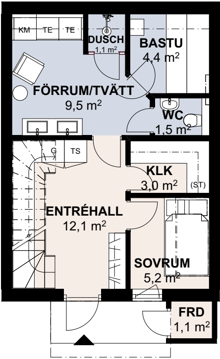
PLAN 1 (KÄLLARE)
