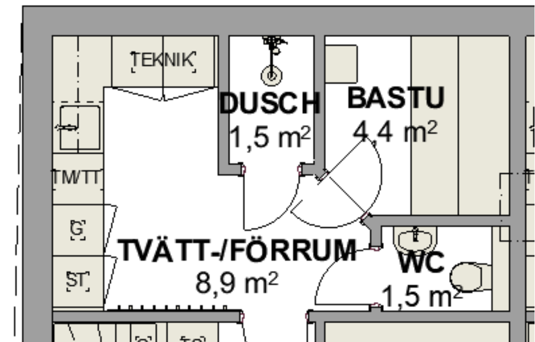
HUSTYP 1 - BADRUM -PLAN
