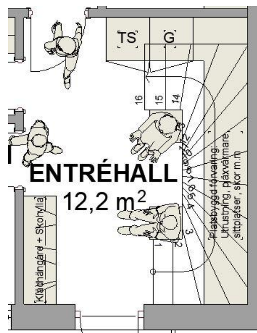
HUSTYP 1 - ENTRÉHALL -PLAN
