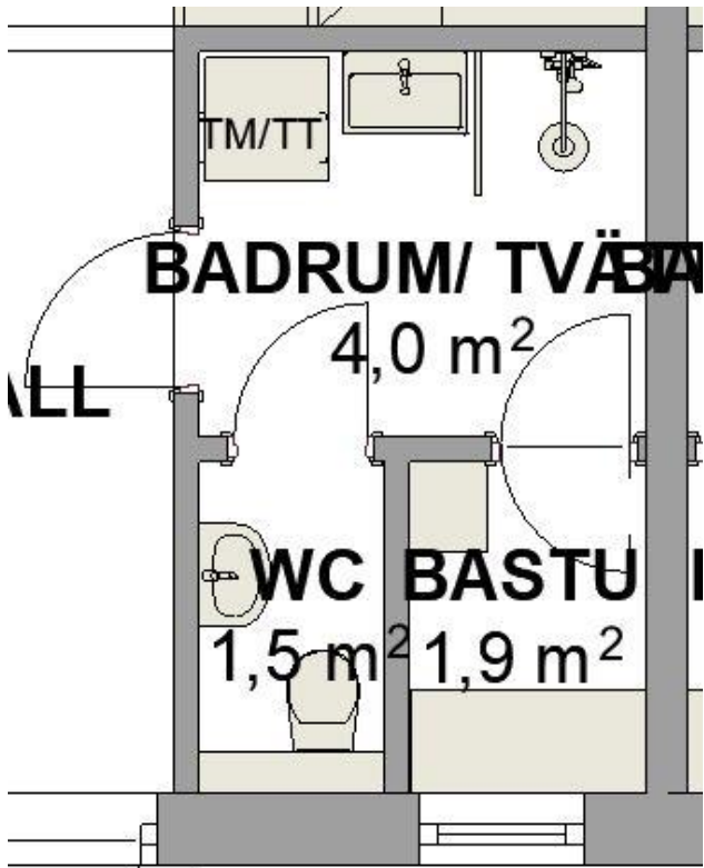
HUSTYP 2 - BADRUM -PLAN
