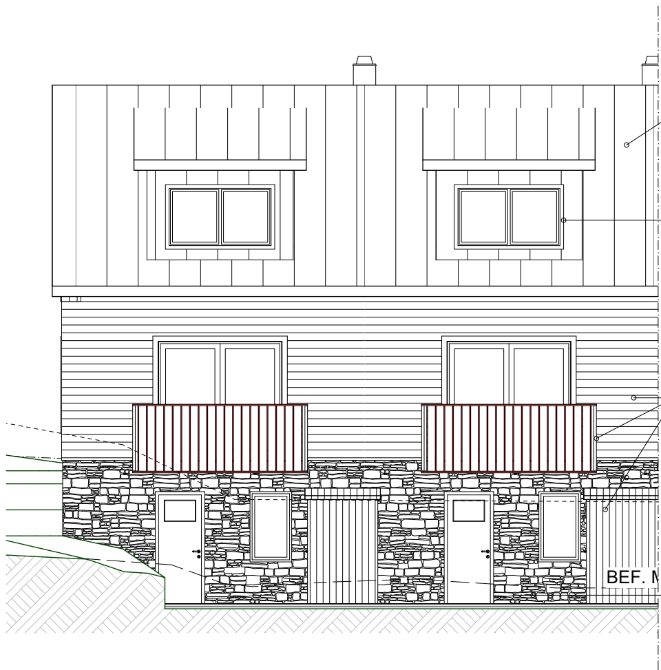
Byggnad A, Fasad mot Ö 1:100
