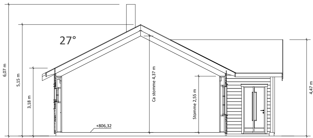
SEKTION B-B 1:100
