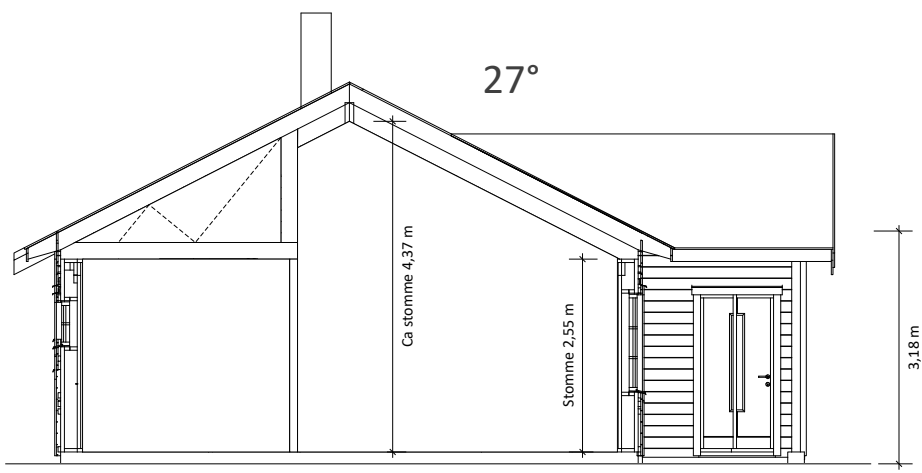
SEKTION C-C 1:100
