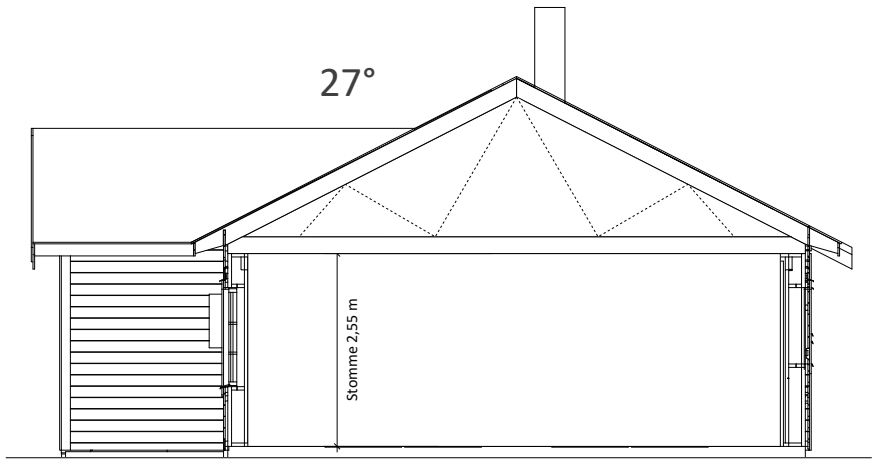
SEKTION A-A 1:100
