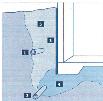
Fuktspär med asfaltstrykning
