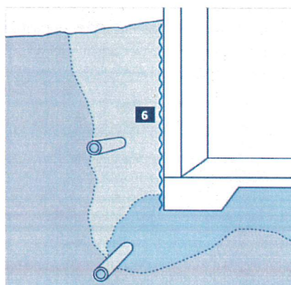
Fuktspär med HD-polyeten
