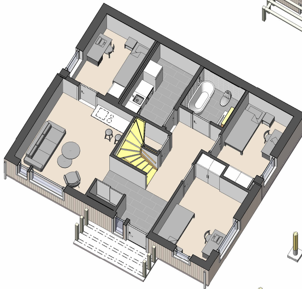
BOTTENVÅNING
