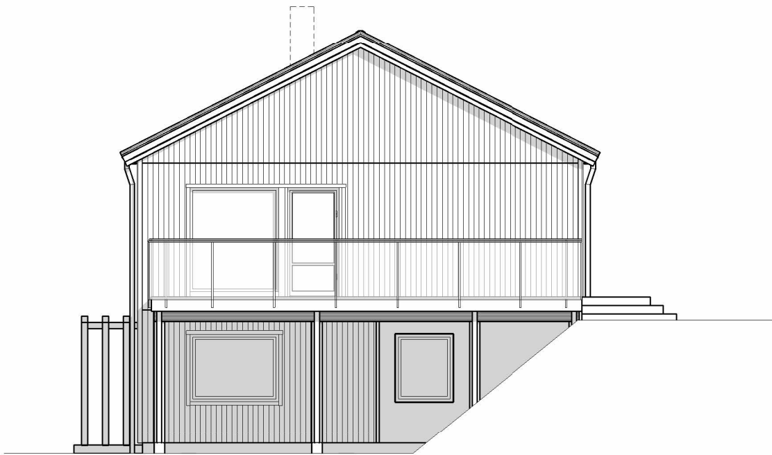
FASAD HÖGERSIDA
