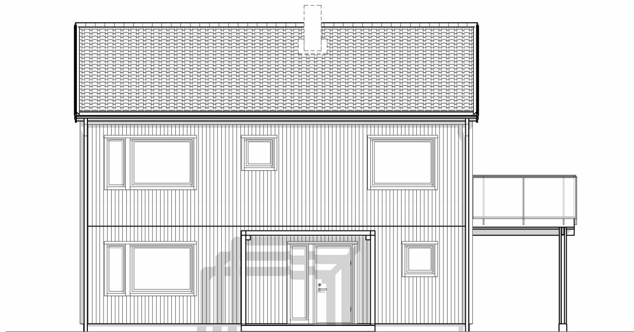
FASAD FRAMSIDA
