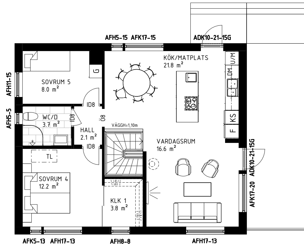
ÖVERVÅNING
