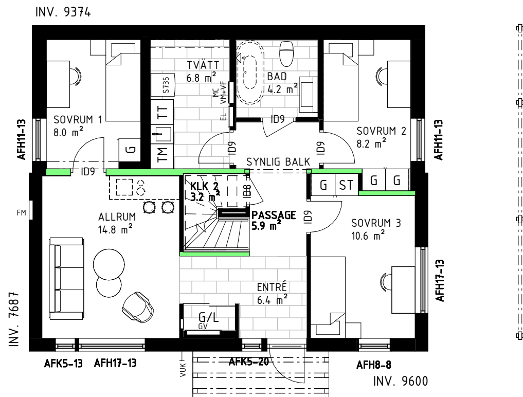
ENTRÉVÅNING
