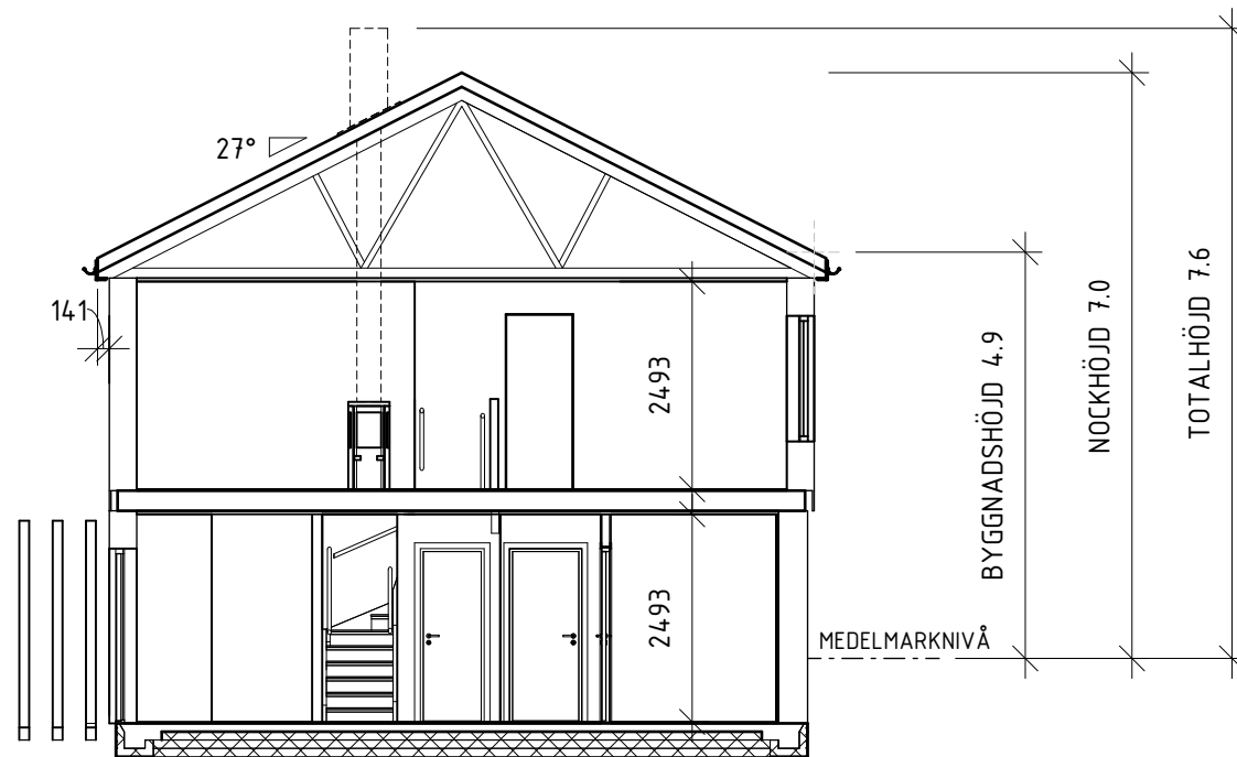
SKÅNETAKFOT SEKTION
